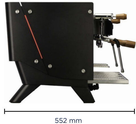
Zijaanzicht
